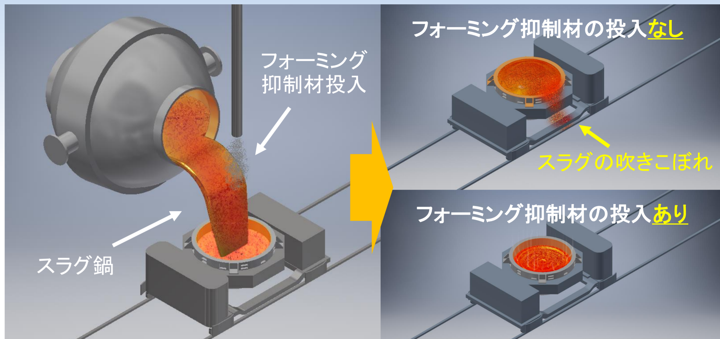
フォーミング抑制材の効果 イメージ
